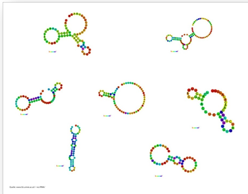
RNA Moleküle
